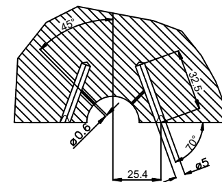
SECTION D-D
